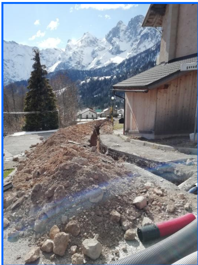
Realizzazione linea interrata distribuzione Passo Cereda –Sagron con eliminazione linea aerea Saresin—Sagron (2022)
