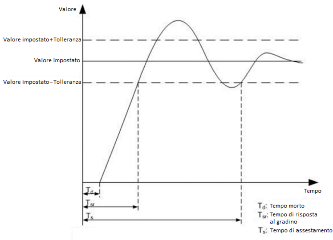
Figura 1 – Risposta al gradino
