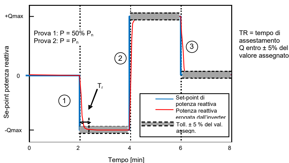
Figura 49 – Misura del tempo di risposta a variazioni a gradino del set-point assegnato per la potenza reattiva
