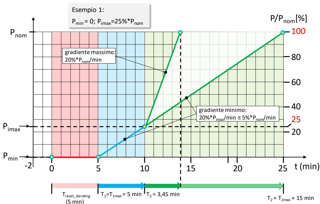
Figura 95 – Funzionamento del regolatore che gestisce il ripristino della erogazione di potenza a valle di un transitorio di sovrافrequenza
