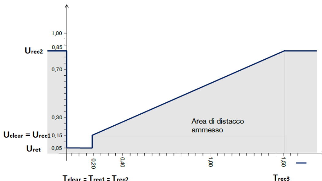
Figura 29 – Profilo di fault-ride-through dei parchi di generazione oltre 11,08 kW
