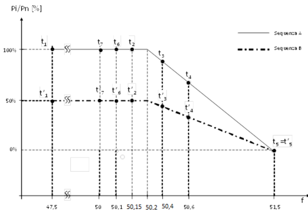
Figura 80 – Curve di limitazione della potenza attiva rispetto alla frequenza per generatori statici (in alto) e per i generatori eolici (in basso)
