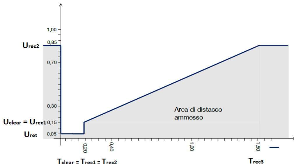
Figura 40 – Profilo di fault-ride-through dei parchi di generazione
