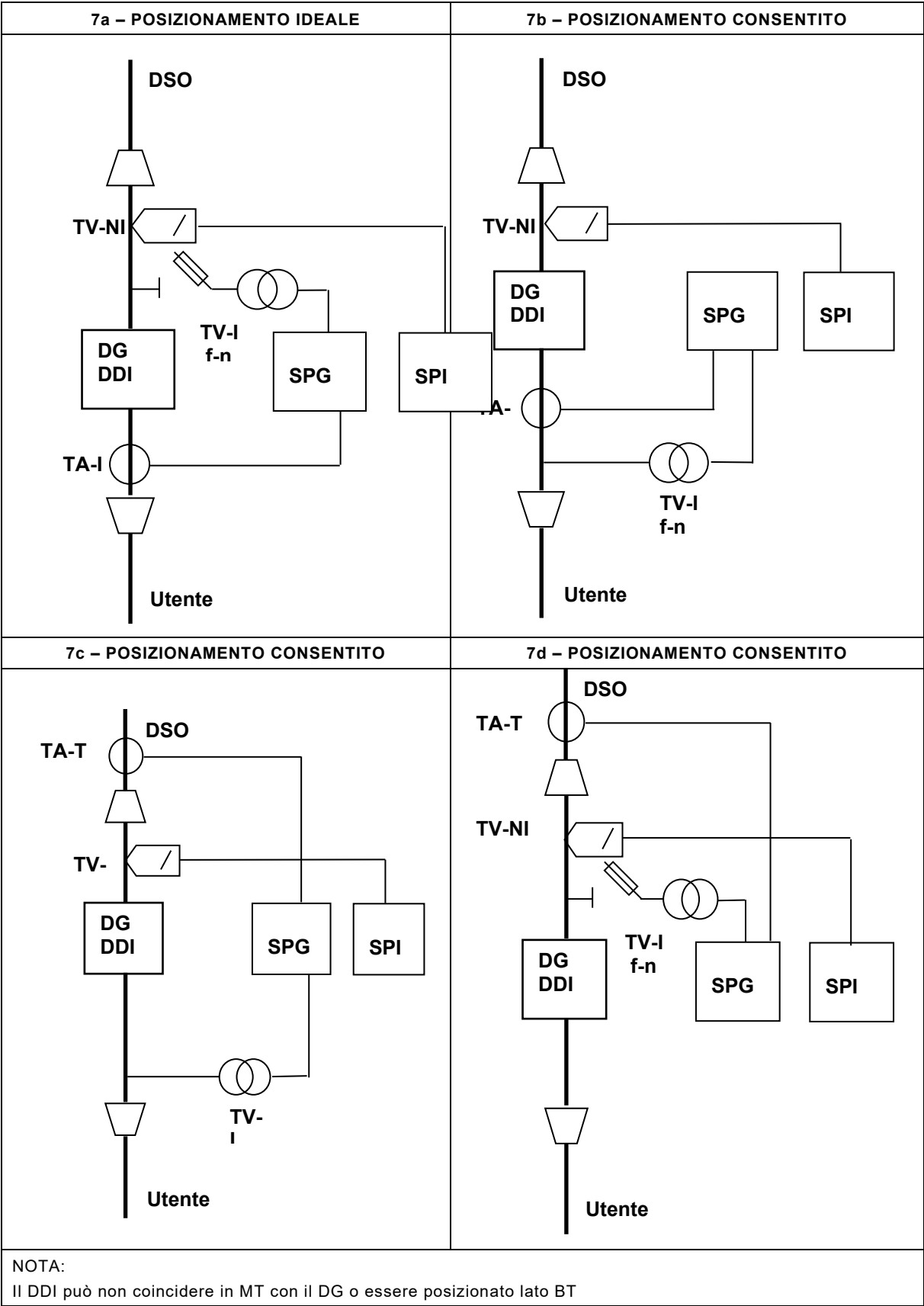
H.7 Schema d'installazione TA-I e TV-I per SPG e TV-NI per SPI, per DG coincidente con DDI (per TO vedi schema H.1)
