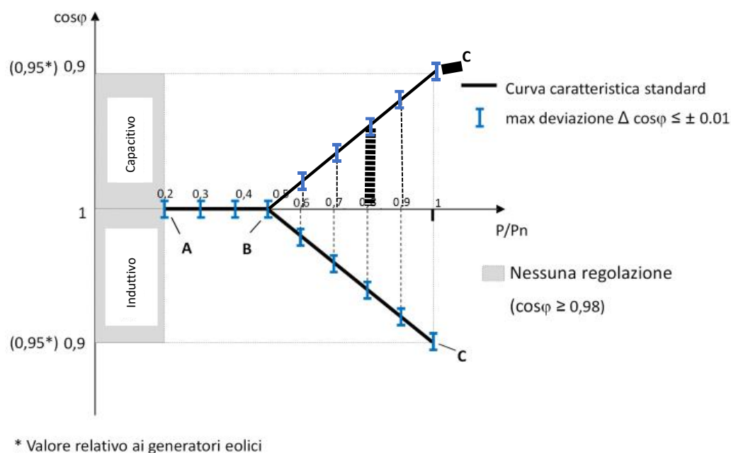
Figura 109 – Variazione del fattore di potenza in funzione della Potenza Attiva
