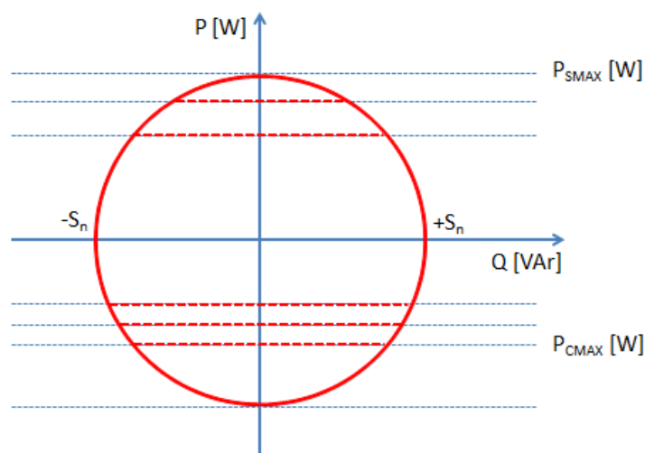
Figura 34 – Combinazione tra capability di un convertitore bidirezionale e accumulatore
